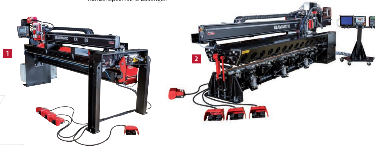
Außenschweißen, Bedienerplattform
