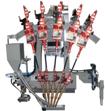
Längsnahtschweißen
